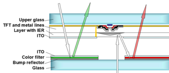
圖 1. 包含前置 TFT 與影像增強層之新型透反式液晶顯示器結構剖面圖。
